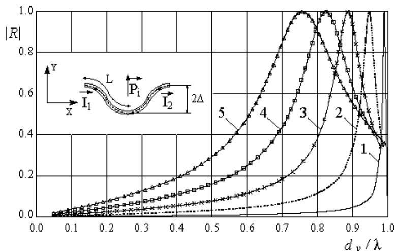
Рис.6. Зависимость модуля коэффициента отражения Н-поляризованной волны от относительной частоты d_y/\lambda для решетки из лент с параметрами d_x = d_y , 2w/d_y = 0.05 , имеющих форму волнистой линии для различных значений \Delta/d_y : кривая 1 - 0.05, кривая 2 - 0.1, кривая 3 - 0.15, кривая 4 - 0.2, кривая 5 - 0.25.
