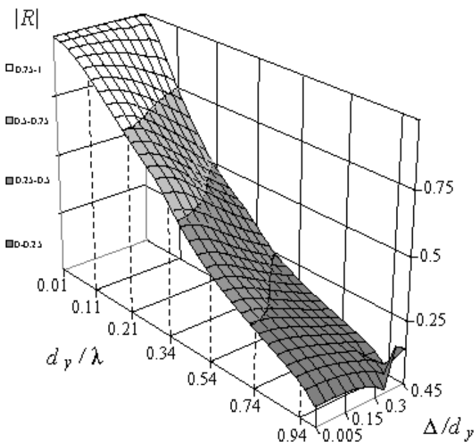
Рис.5. Зависимость модуля коэффициента отражения Е-поляризованной волны от относительной частоты d_y/\lambda и максимального отклонения линии от средней прямой для решетки из лент имеющих пилообразную форму с параметрами d_x = d_y , 2w/d_y = 0.05 .
