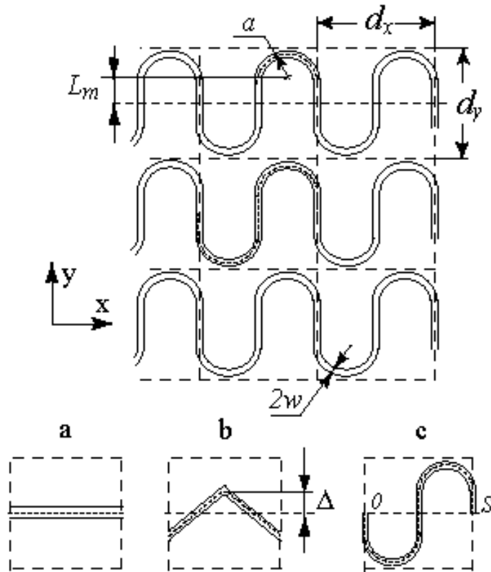
Рис.1 Плоская периодическая в двух направлениях решетка и некоторые варианты геометрии периода
