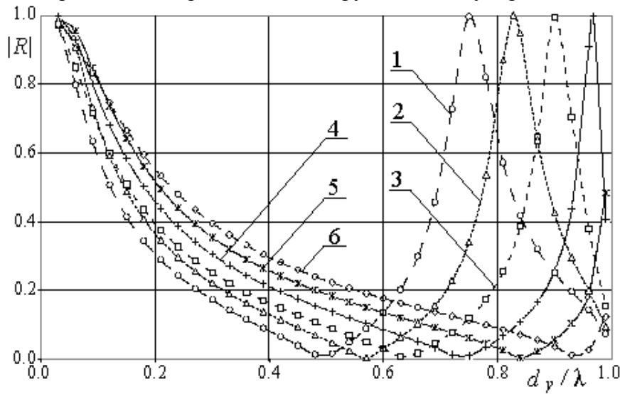
Рис.4. Зависимость модуля коэффициента отражения Е-поляризованной волны от относительной частоты d_y/\lambda для решетки из лент с параметрами d_x = d_y , 2w/d_y = 0.05 , имеющих форму меандра для различных значений L_m/d_y : кривая 1 – 0.25, кривая 2 – 0.2, кривая 3 – 0.15, кривая 4 – 0.1, кривая 5 – 0.05, кривая 6 – 0.0.
