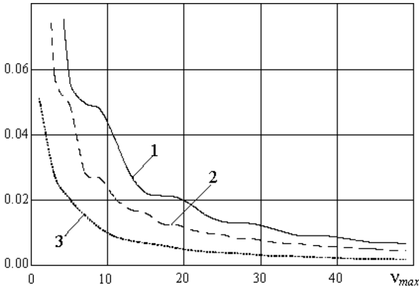
Рис.2. Зависимость относительной ошибки вычисления модуля коэффициента отражения решетки из прямых лент от v_{max} : d_x = d_y , d_y/\lambda = 0.5 , 2w/d_y = 0.1 (кривая 1), 2w/d_y = 0.2 (кривая 2), 2w/d_y = 0.4 (кривая 3).
